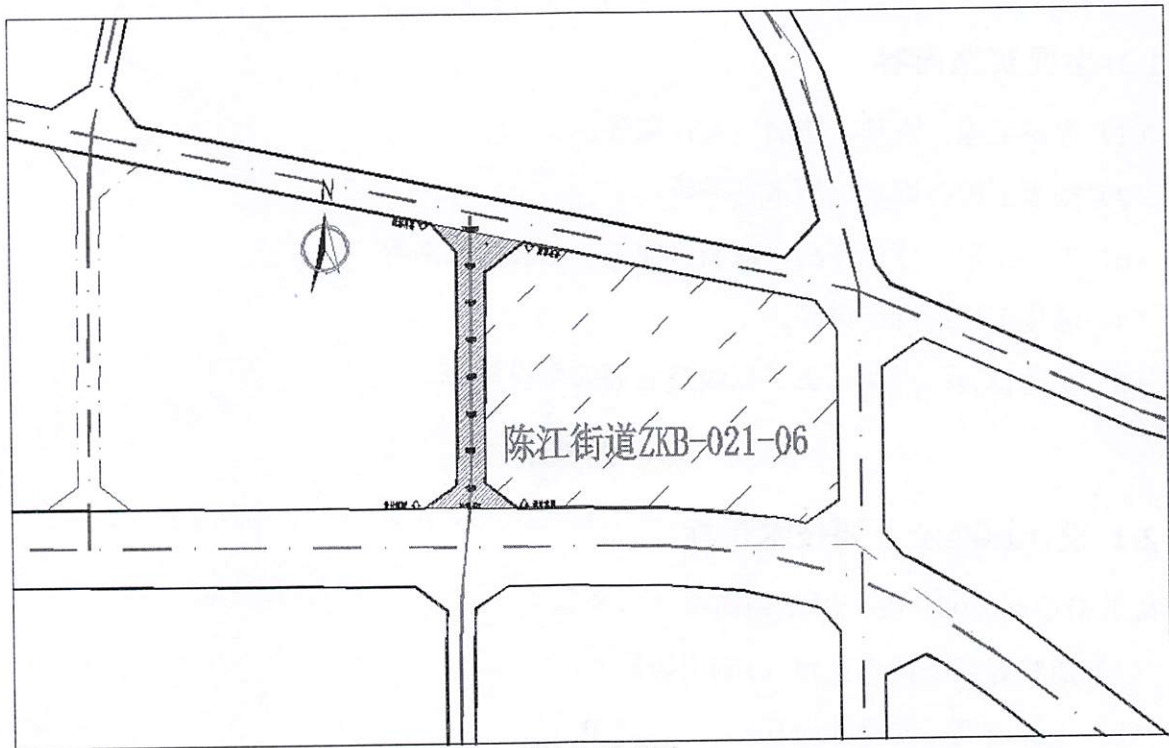
项目总平面图
