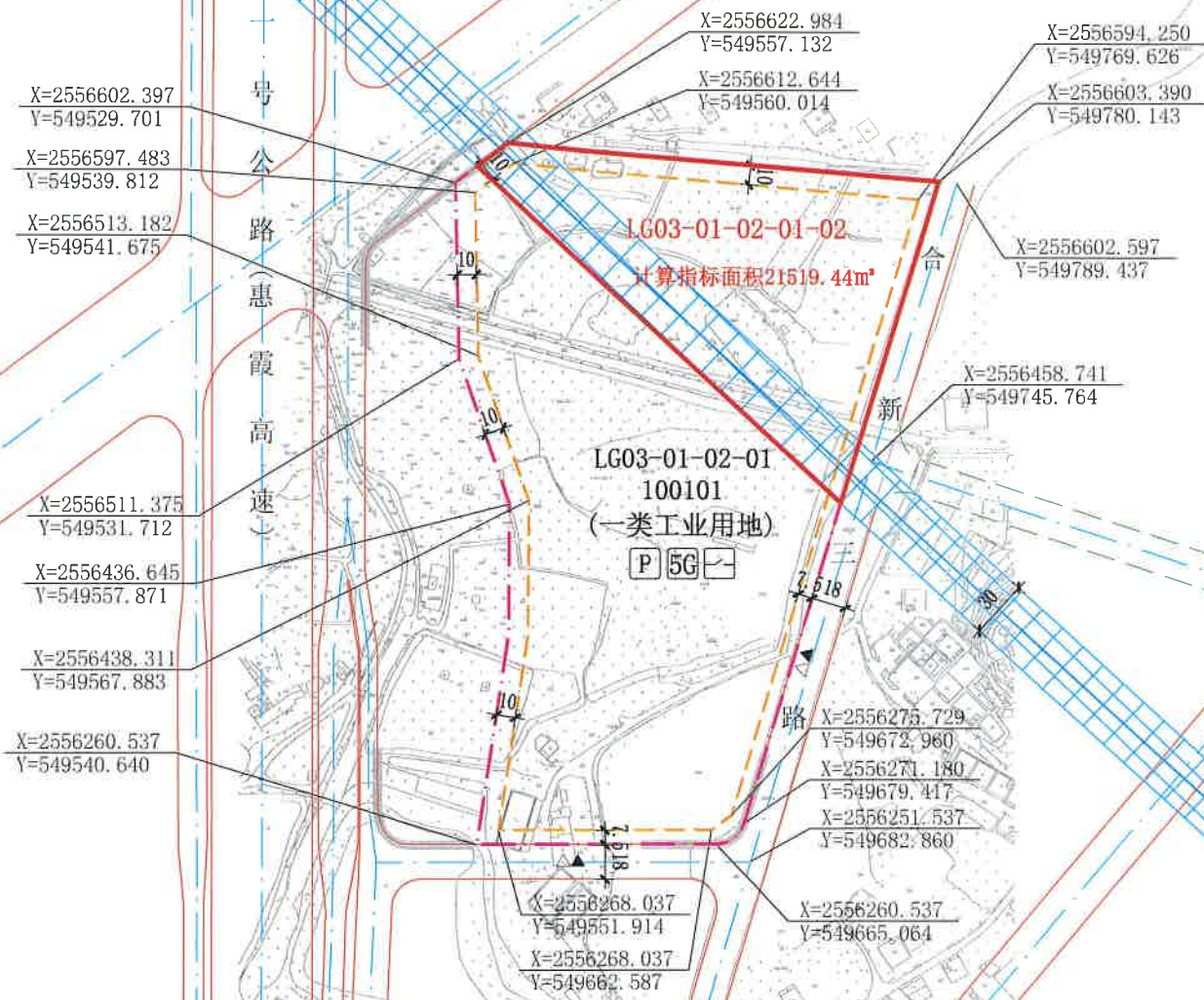
规划控制图
