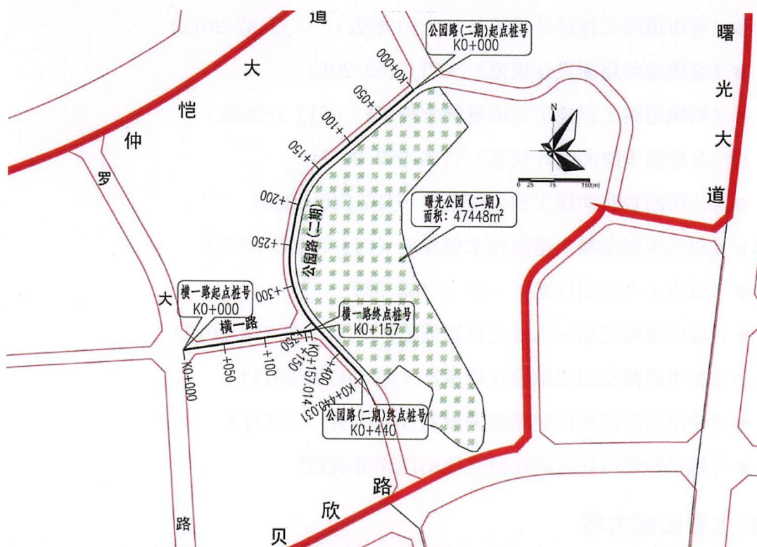
项目总平面图
