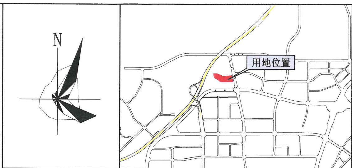
风玫瑰
