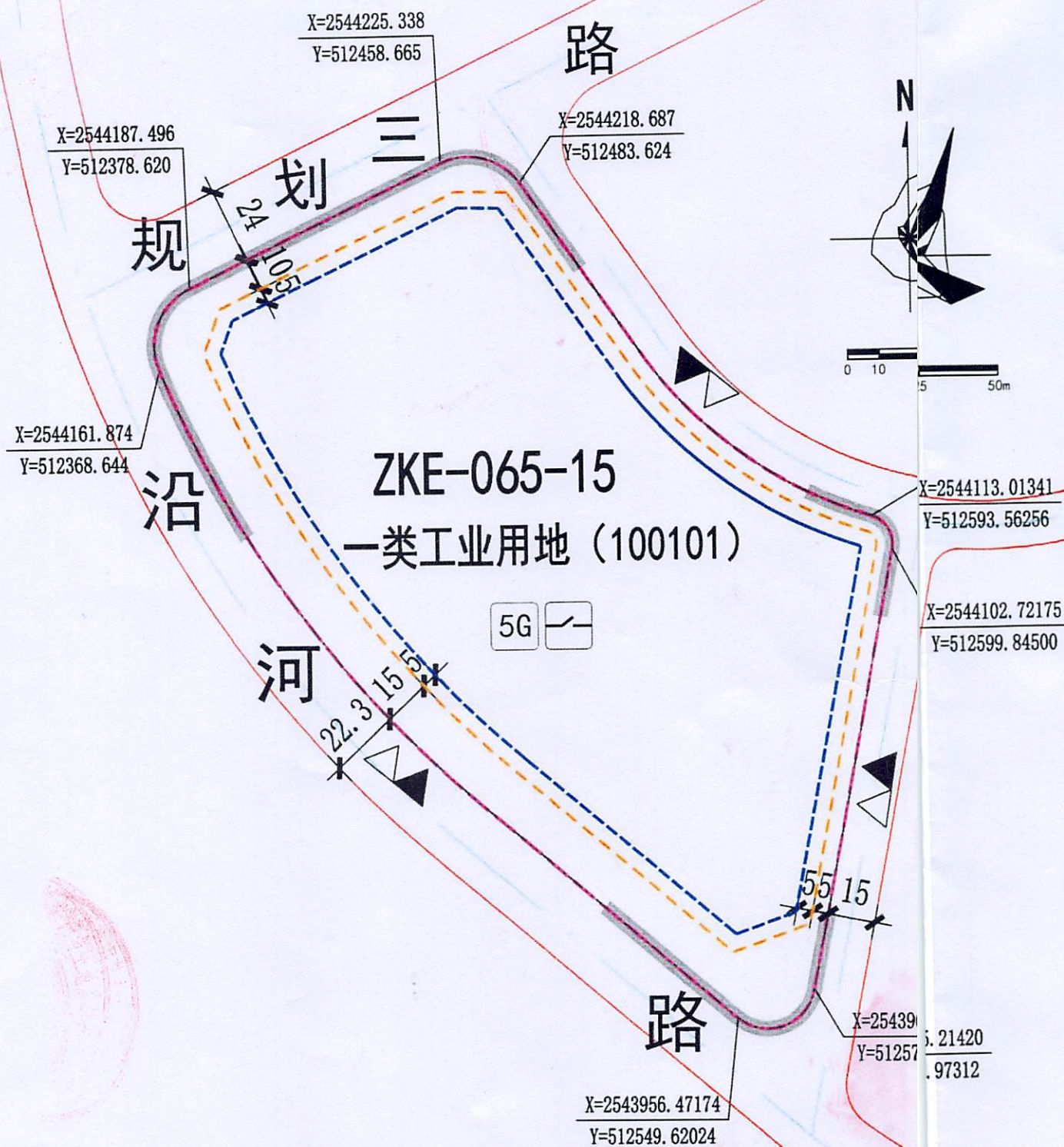
规划控制图
