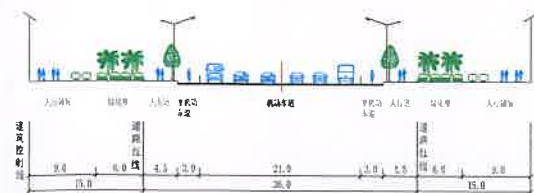
B1-B1道路横断面图
